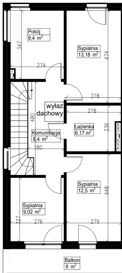
Rzut 1 piętra
